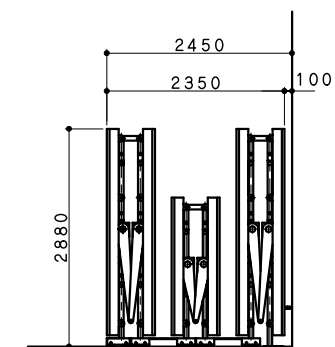
収納側面図 (128帖 公式サイズ)
