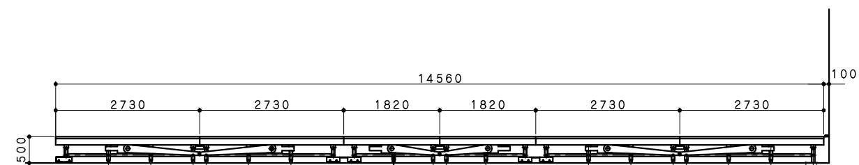
展開側面図 (128帖 公式サイズ)
