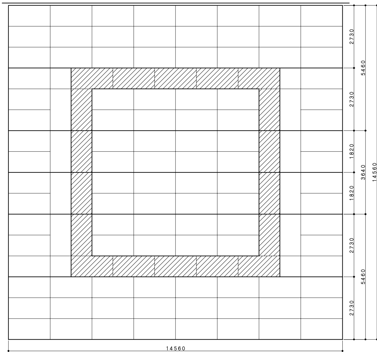
平面図 (128帖 公式サイズ)
