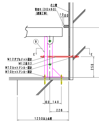
A部固定スタンド詳細図
