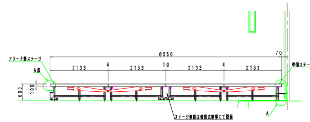
使用時側面図
