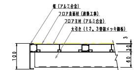
B部フローアース断面図
