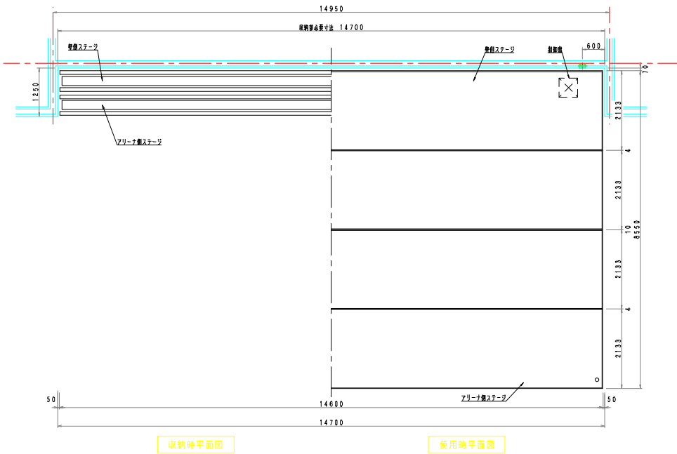
収納時平面図
