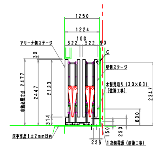
収納時側面図
